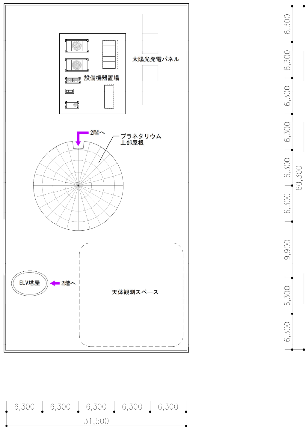
屋上階平面図
