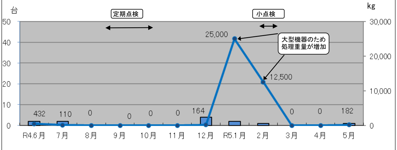
変圧器類の処理台数及び処理重量の推移(直近1年間の各月)
