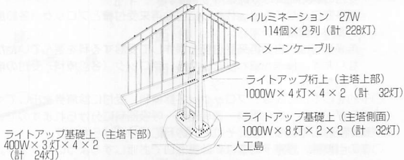
白鳥大橋ライトアップ・イルミネーション概要図
