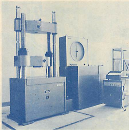
◀万能材料試験機(50t) 金属材料等の引張り・曲げ・ 圧縮などの試験検査に
