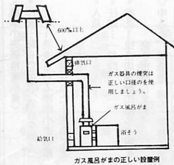
ガス風呂がまの正しい設置例
