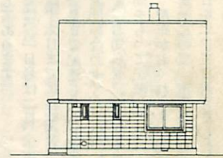
東側立面図
