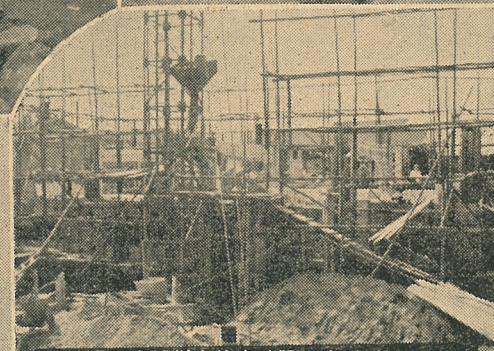
⑨ 千才町店舗併存住宅建設工事（鉄筋コンクリート四階建）一・二階は店舗・三・四階は住宅。
