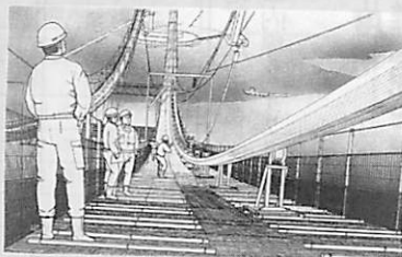
ケーブルストランドの架設工事
