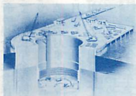
④連続壁の内部を掘削し、上からコンクリートを巻く
