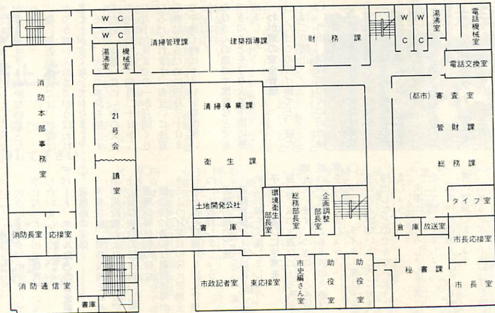
2階平面図
